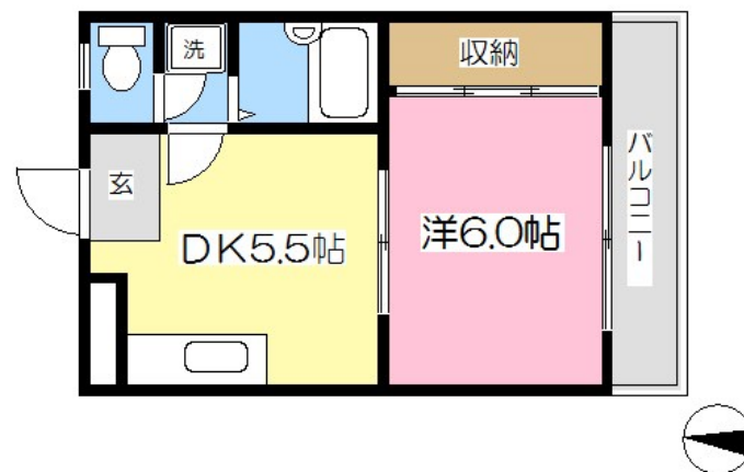
【間取り図】
