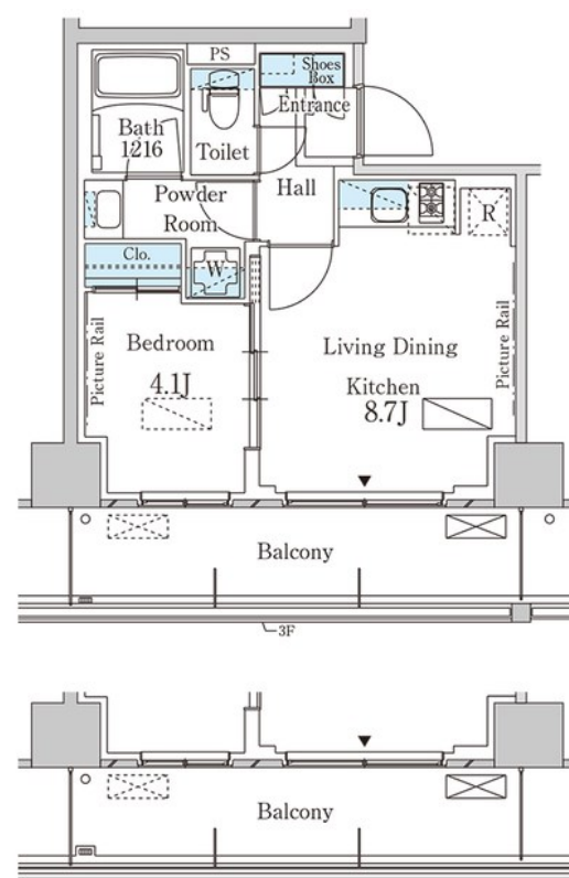
【間取り図】
